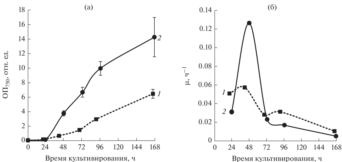
Рис. 4. Зависимость роста Chlorella sp. IPPAS C-1210 от интенсивности освещения при температуре 30^\circ\text{C} и подаче ГВС с концентрацией CO_2 1.5–1.8%. Ростовые кривые – (а); удельная скорость роста – (б). 1 – 100 \text{ мкмоль}/(\text{м}^2 \cdot \text{с}) ; 2 – 500 \text{ мкмоль}/(\text{м}^2 \cdot \text{с}) . Показаны средние значения и стандартные отклонения по трем повторностям.
