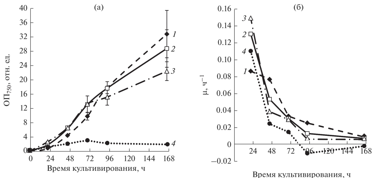
Рис. 3. Зависимость роста C. sorokiniana IPPAS C-1 от температуры при подаче ГВС с концентрацией CO_2 1.5–1.8% и постоянном освещении 500 \text{ мкмоль}/(\text{м}^2 \cdot \text{с}) . Ростовые кривые – (а); удельная скорость роста – (б) 1 – 26^\circ\text{C} ; 2 – 31^\circ\text{C} ; 3 – 36^\circ\text{C} ; 4 – 41^\circ\text{C} . Показаны средние значения и стандартные отклонения по трем повторностям.
