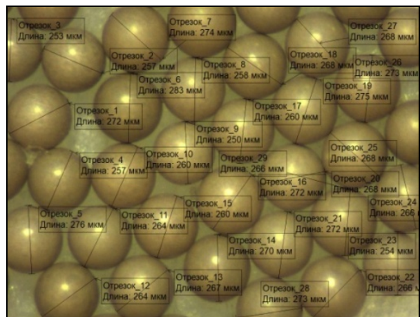
Гашково, 2017 г., (264,45 \pm 0,68) мкм
