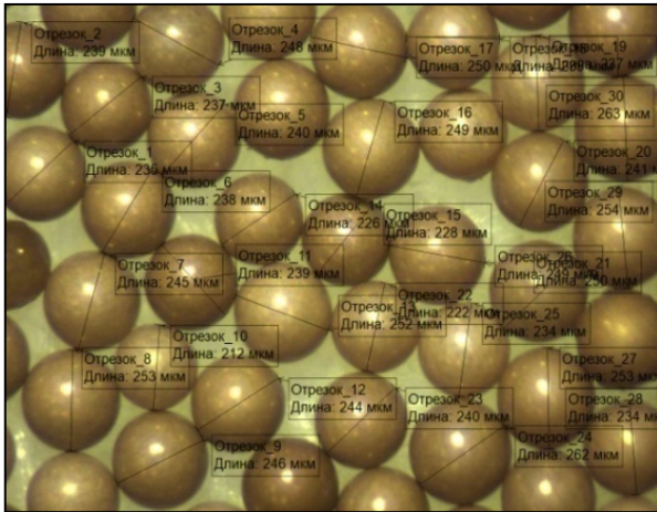
Большое Яровое, 2017 г., (243,52 \pm 0,62) мкм
