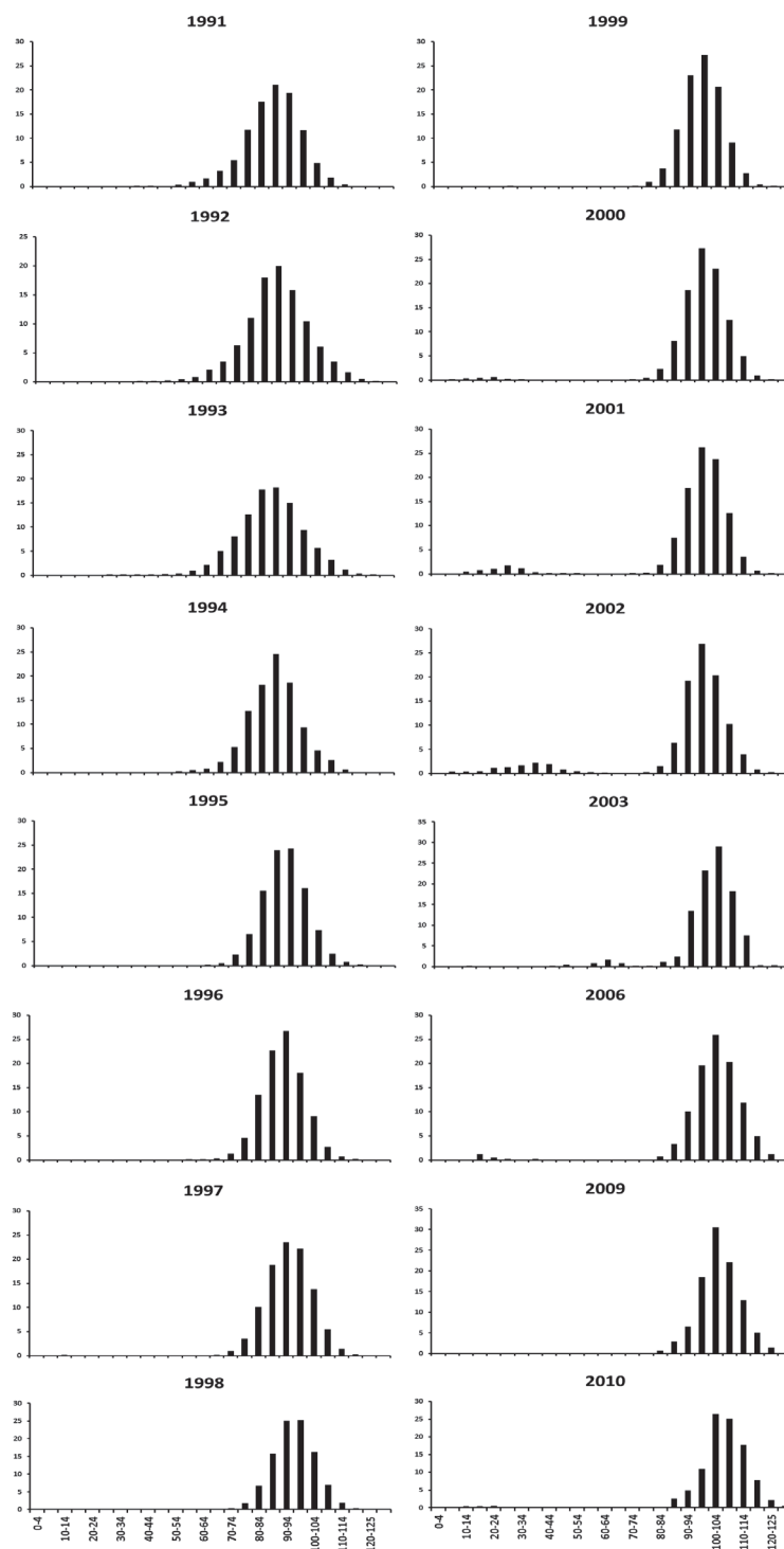
Рис. 3. Размерный состав гребешка на северо-восточном участке Святоносского поселения в 1991–2010 гг.
