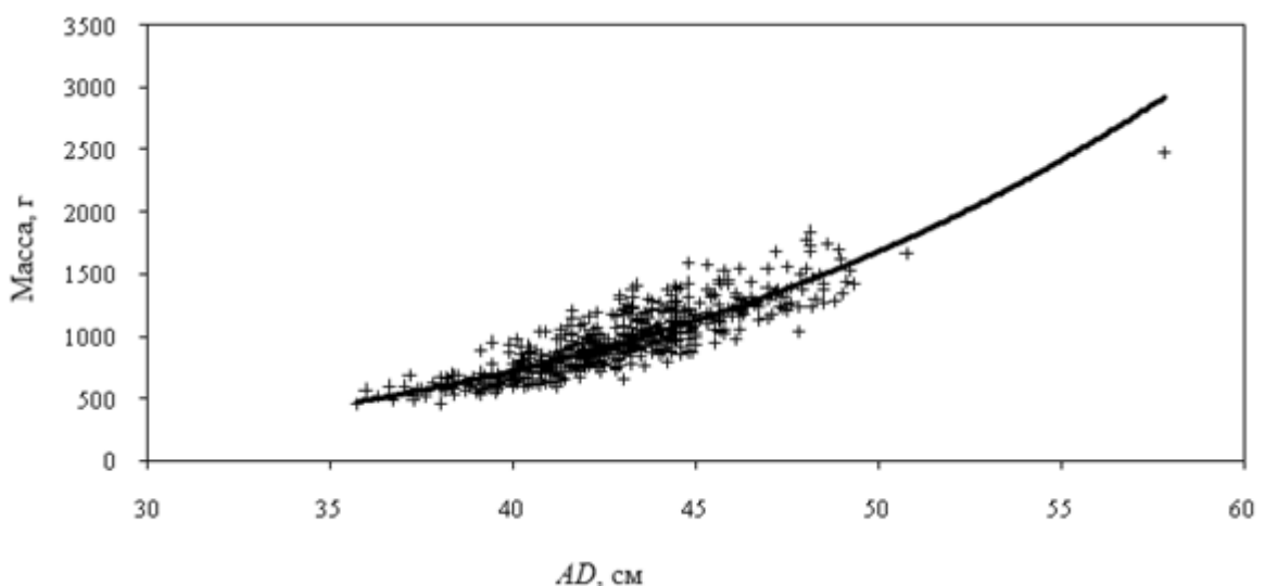
Рис. 1. Зависимость массы особей Coregonus autumnalis р. Индигирка от длины AD ( y = 0.000x^{3.814} , R^2 = 0.765 ).
