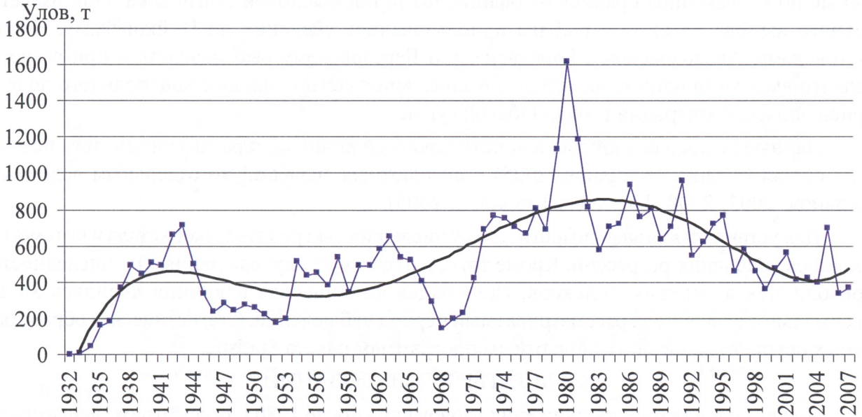
Рис. 1. Динамика уловов чира бассейна реки Обь. Fig. 1. The dynamics of chirs catches of the Ob basin.
