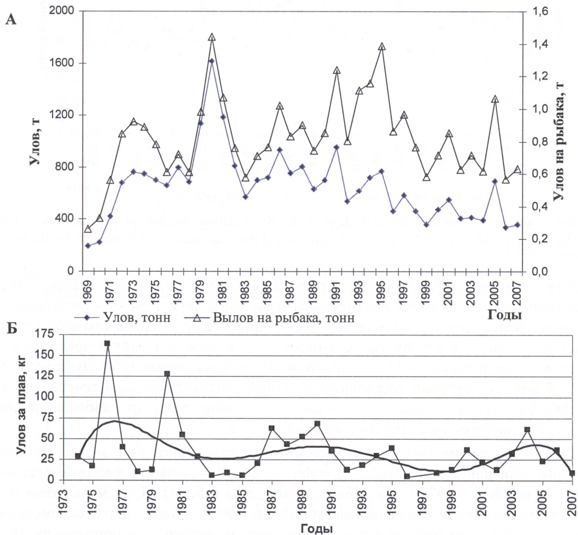
Рис. 2. Динамика уловов чира на стандартизированное усилие. А – улов на одного рыбака; Б – улов за один контрольный плав в период вонзевой миграции рыб (сети 300 м, ячей 60-70 мм).
