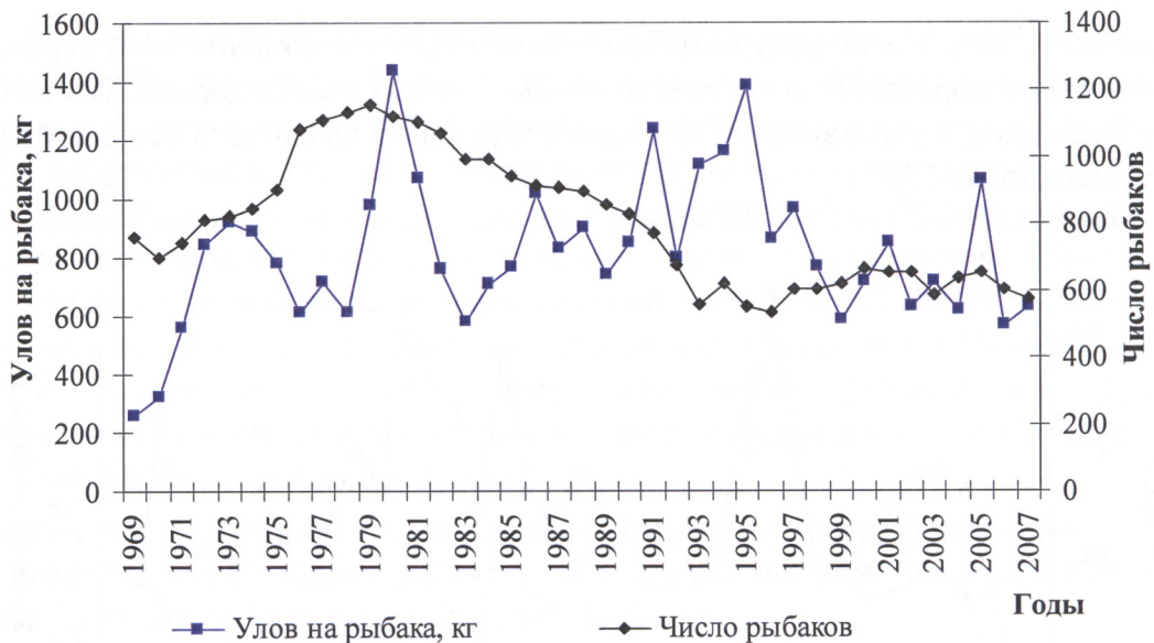
Рис. 3. Динамика улова чира на одного рыбака и общей численности рыбаков за период 1969-2007 гг. Fig. 3. The dynamics of chir catches on one fisherman and the total number of fishermen for the period of 1969-2007.
