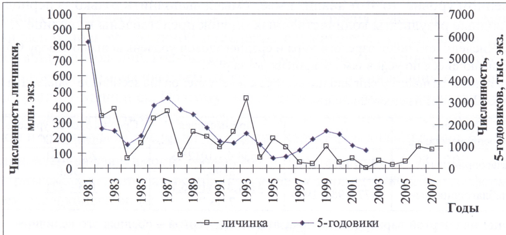
Рис. 5. Динамика численности личинки в год t и 5-годовиков чира в год t-5 . Fig. 5. The dynamics of larva number per year t and 5 years individuals of chir per year t-5 .
