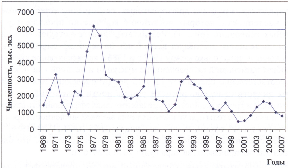
Рис. 4. Динамика численности пятигодовалых особей чира за период 1969-2007 гг. Fig. 4. The dynamics of the number of 5 years individuals chir for the period 1969-2007.
