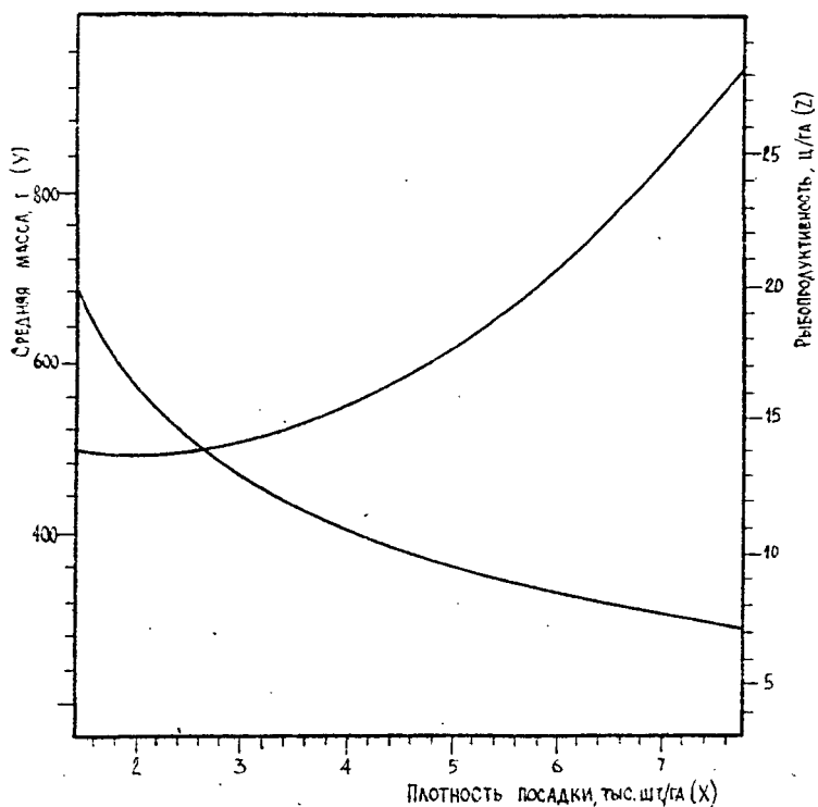
Рис.4. Зависимость средней массы ( y ) и рыбопродуктивности ( z ) от плотности выращивания двухлетков для условий рыбхоза "Лаква"
