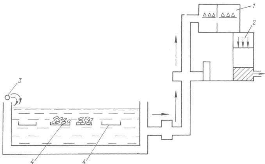
Рис. 31. Схема очистительного устричного танка с рециркуляционной системой водо> подачи [208]:
