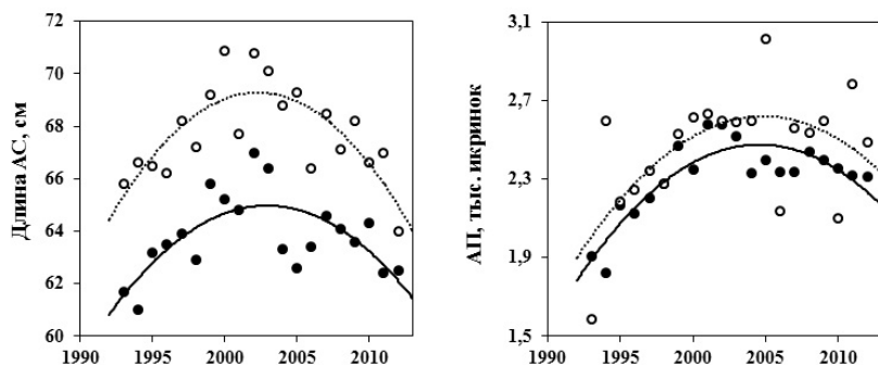
Рис. 3.10. Изменения длины тела и плодовитости у четырехлеток (темные символы, сплошная линия) и пятилеток (светлые символы, пунктир) кеты в р. Илюшина в 1993–2012 гг.
