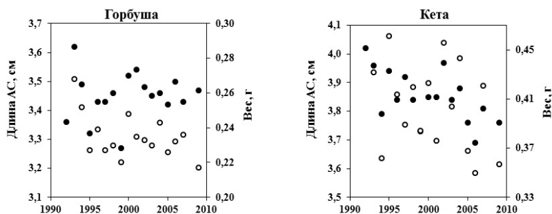
Рис. 3.12. Межгодовые изменения длины (темные символы) и веса (светлые символы) тела покатной молоди горбуши и кеты в р. Илюшина в 1992–2009 гг.
