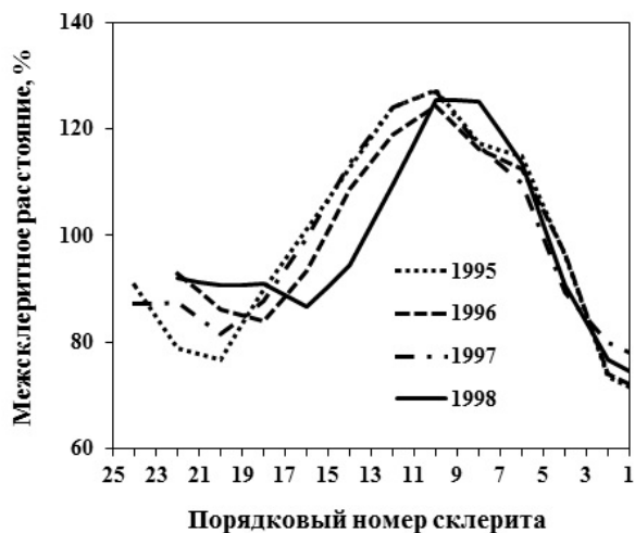
Рис. 3.5. Склеритогаммы ПГЗ чешуи горбуши позднего хода в р. Илюшина на о-ве Кунашир в 1995–1998 гг.
