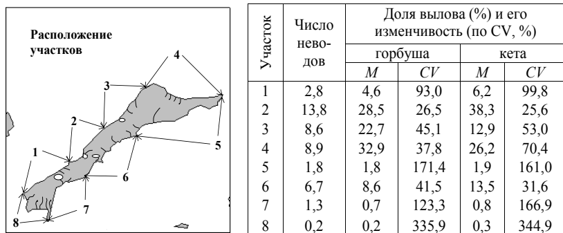
Рис. 3.3. Количество ставных неводов и доля вылавливаемой горбуши и кеты на разных участках побережья о-ва Кунашир в среднем за период 2001–2012 гг.
