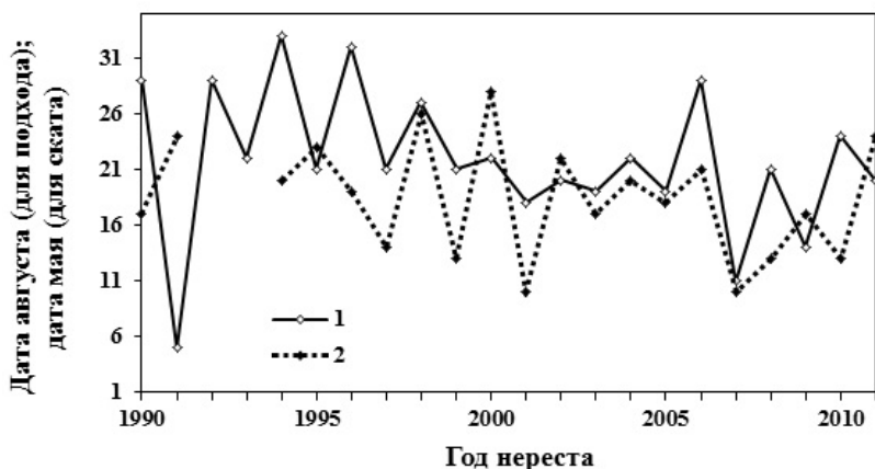
Рис. 3.14. Изменения средних сроков подхода рыб (по датам 50-процентного промыслового вылова) и последующего ската молоди (по датам наступления 50-процентной кумуляты количества скатывавшихся мальков) у разных поколений горбуши о-ва Кунашир.
