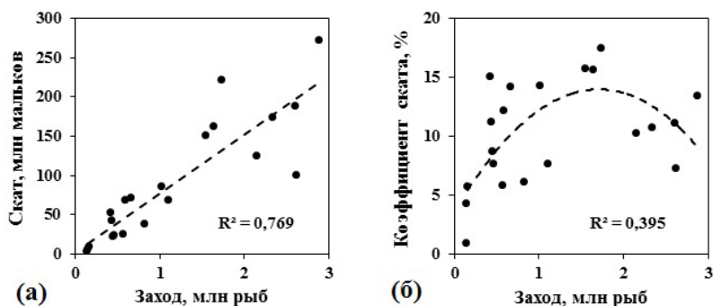
Рис. 3.16. Изменения численности покатной молоди (а) и эффективности воспроизводства в пресноводном периоде жизни (б) в связи с численностью производителей горбуши в реках о-ва Кунашир в 1990–1991, 1994–2012 гг.
