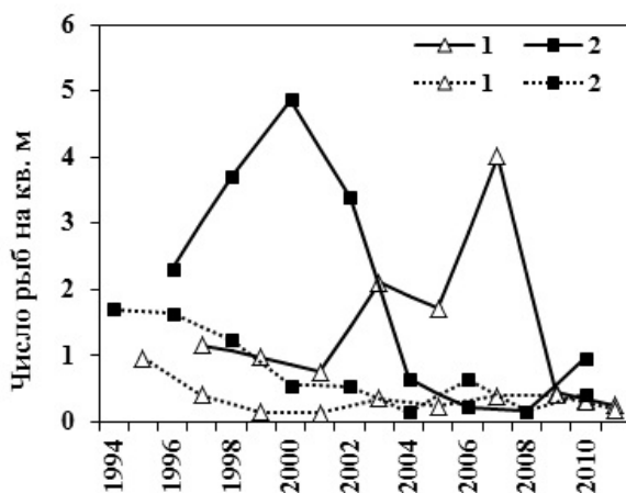
Рис. 3.4. Заполнение нерестилищ горбушей в р. Илюшина в первой половине сентября (сплошная линия) и в первой декаде октября (пунктир) в нечетные (1) и четные (2) 1994–2011 гг.
