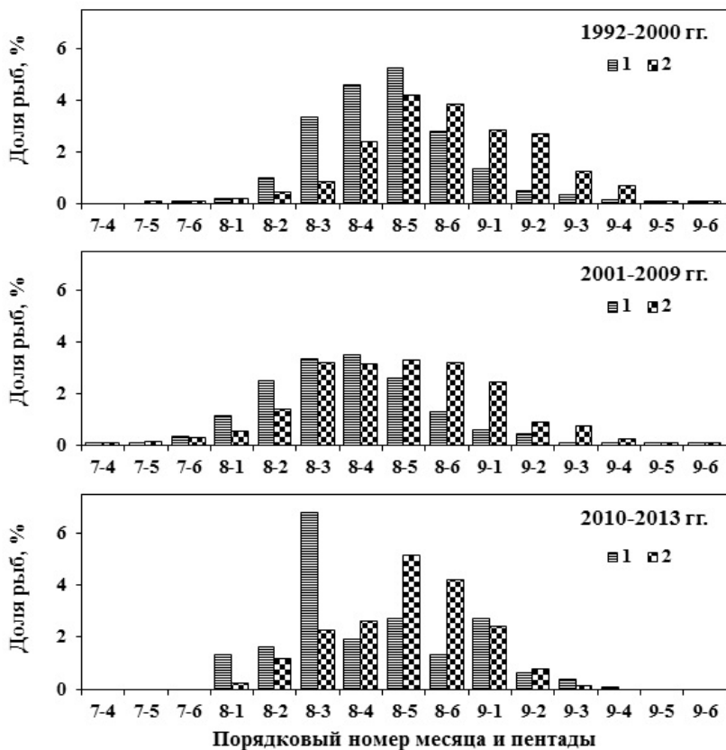
Рис. 4.2. Динамика среднесуточных по пентадам уловов горбуши в водах о-ва Кунашир в нечетные (1) и четные (2) годы разных периодов (1992–2000, 2001–2009 и 2010–2013 гг.).
