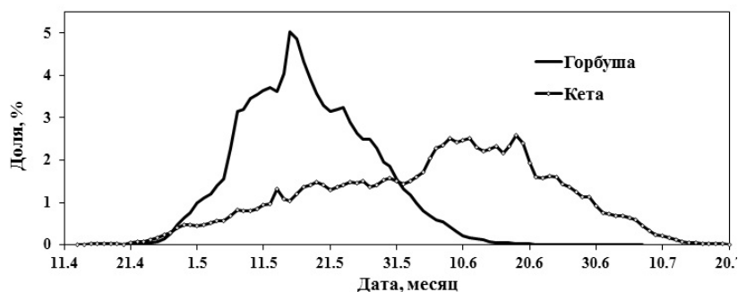
Рис. 3.11. Динамика покатной миграции молоди горбуши и кеты в р. Илюшина в среднем за 1991–1992, 1995–2013 гг.
