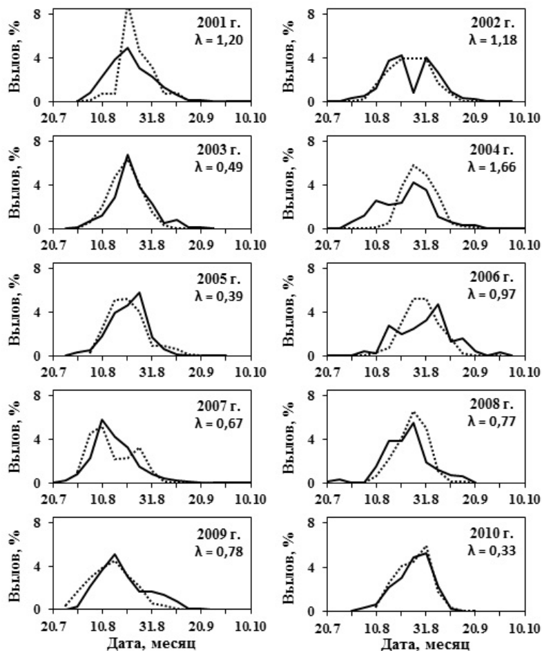
Рис. 3.15. Динамика промысловых уловов горбуши в прибрежье о-ва Кунашир в 1991, 1994–2010 гг. (сплошная линия) и динамика последующей покатной миграции молоди этих поколений в р. Илюшина (пунктирная линия): совмещение распределений по дате 50-процентной кумуляты.
