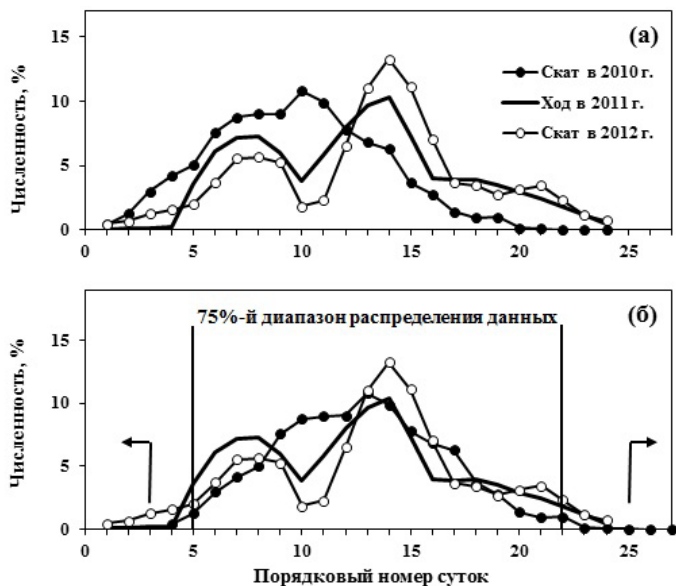
Рис. 4.8. Совмещение распределений динамики подходов горбуши и покатной миграции молоди: (а) – исходные распределения, (б) – совмещение распределений; стрелками обозначены удаляемые фрагменты распределений (пояснения см. в тексте).
