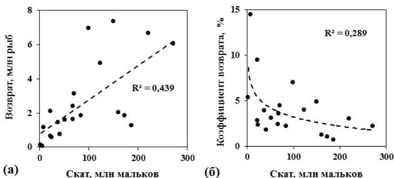
Рис. 3.17. Изменения численности возврата (а) и выживаемости рыб в течение морского периода жизни (б) в связи с численностью покатной молоди соответствующих поколений горбуши о-ва Кунашир.
