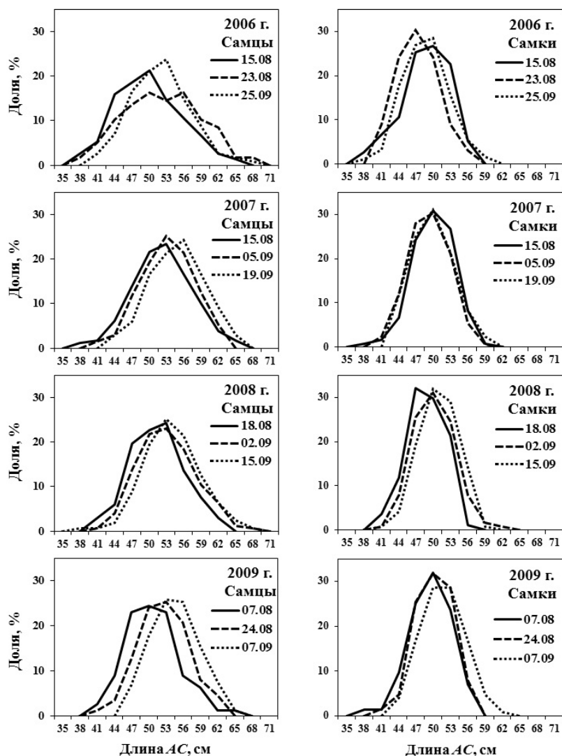
Рис. 4.3. Распределения по длине тела самцов и самок горбуши в разных пробах, собранных в р. Илюшина в 2006–2009 гг.
