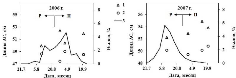
Рис. 4.6. Динамика уловов и длины тела самцов и самок горбуши на о-ве Кунашир в 2006, 2007 гг.: 1 – длина самцов, 2 – длина самок, 3 – суточный вылов, стрелками обозначено время смены ранней формы (P) на позднюю форму (II).
