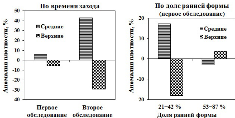
Рис. 4.4. Изменения плотности заполнения горбушей средних и верхних нерестилищ в р. Илюшина в зависимости от времени хода и соотношения темпоральных форм в 1995–2010 гг.
