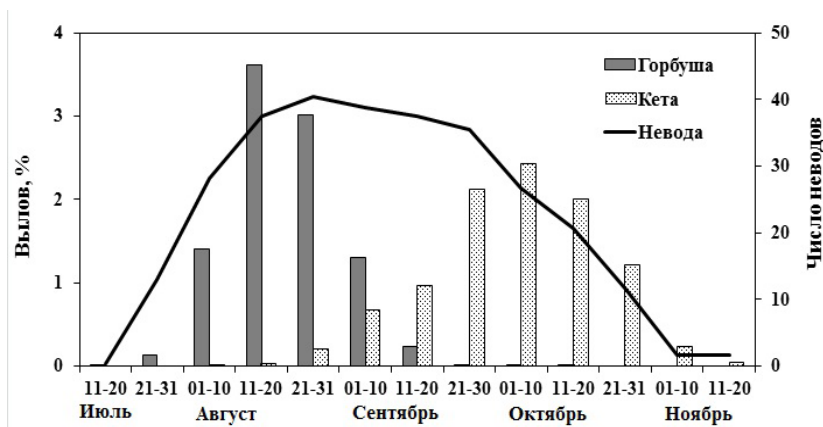
Рис. 3.2. Динамика среднесуточных по декадам уловов горбуши и кеты и количества ставных неводов на о-ве Кунашир в 2001–2013 гг.
