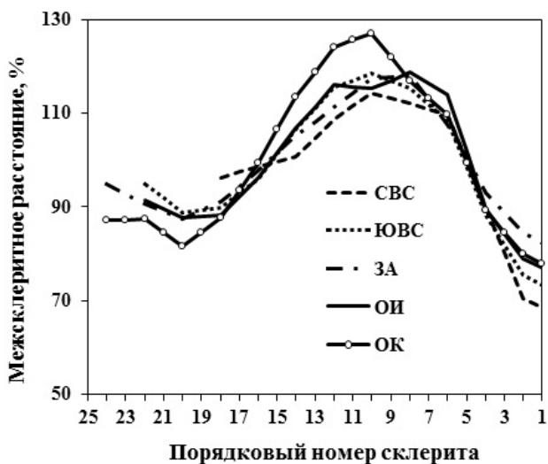
Рис. 3.6. Склеритогаммы ПГЗ чешуи горбуши позднего хода в разных районах в 1997 г.: СВС – северо-восточный Сахалин, ЮВС – юго-восточный Сахалин, ЗА – зал. Анива, ОИ – о-в Итуруп, ОК – о-в Кунашир.
