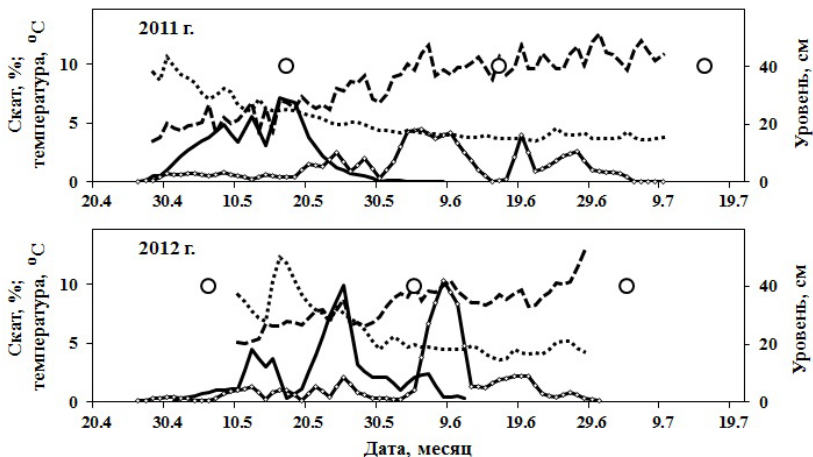
Рис. 3.13 в. Динамика покатной миграции молоди горбуши (1) и кеты (2), температуры (3) и уровня воды (4) в р. Илюшина в разные годы: 5 – дата полнолуния.
