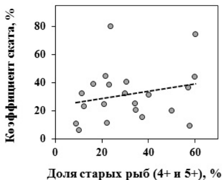
Рис. 3.20. Изменения эффективности нереста кеты с возрастом родителей в 1990–1991, 1994–2012 гг. в р. Илюшина.
