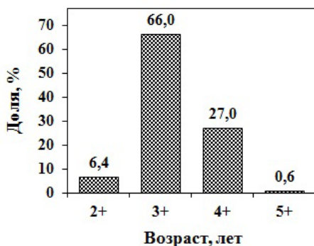
Рис. 3.19. Соотношение рыб разного возраста в возвратах поколений кеты в р. Илюшина в среднем за годы наблюдений.
