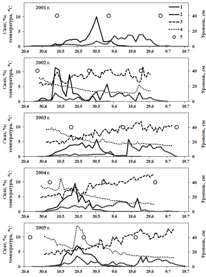
Рис. 3.13 а. Динамика покатной миграции молоди горбуши (1) и кеты (2), температуры (3) и уровня воды (4) в р. Илюшина в разные годы: 5 – дата полнолуния.
