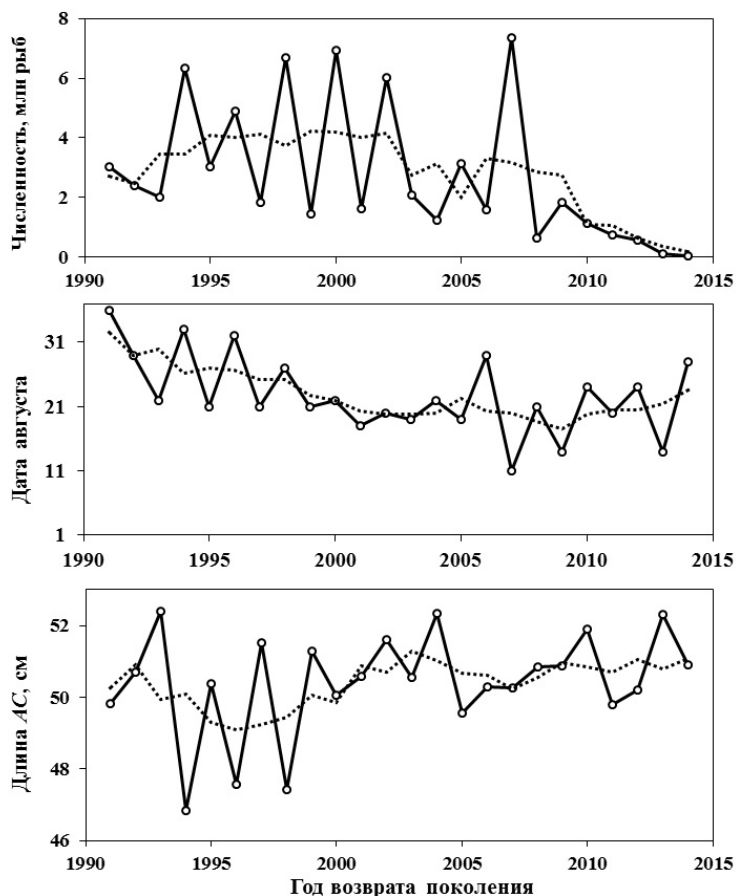
Рис. 3.8. Изменения численности, сроков подхода (по дате достижения 50-процентного вылова) и длины тела у горбуши о-ва Кунашир в 1991–2014 гг.: сплошная линия с символами – фактические значения, пунктирная линия – скользящая средняя (по четырём смежным значениям).
