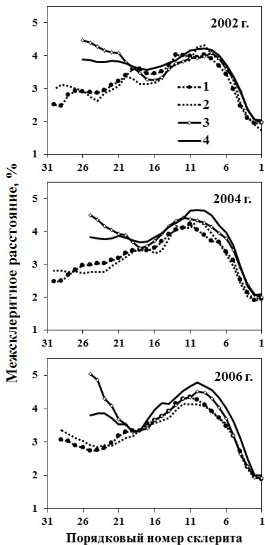
Рис. 5.2. Склеритограммы первой годовой зоны роста чешуи кеты островов Кунашир (1 и 2) и Итуруп (3 и 4), пойманной в 2002, 2004, 2006 гг.: 1 и 3 – речная кета, 2 и 4 – озерная кета; отсчет склеритов – от первого годового кольца к центру чешуи.
