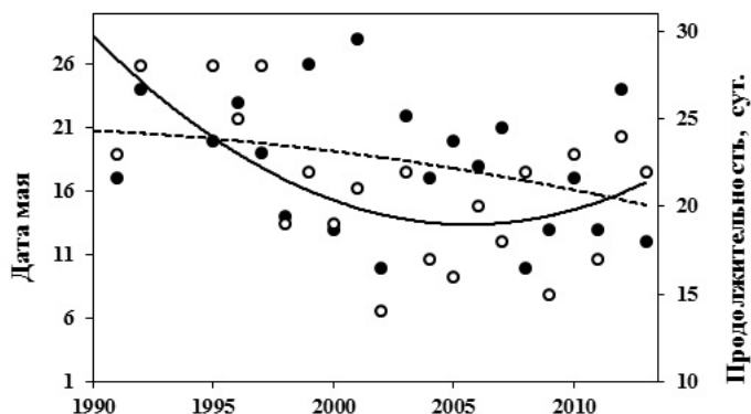
Рис. 4.5. Изменения даты наступления середины (темные символы, пунктирная линия) и продолжительности периода массового ската (светлые символы, сплошная линия) молоди горбуши в р. Илюшина в 1991–1992, 1995–2013 гг.
