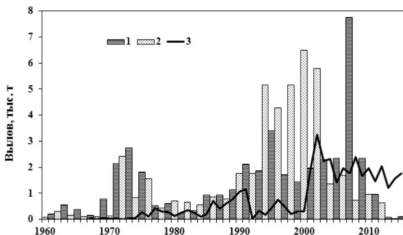
Рис. 3.1. Уловы горбуши поколений нечетных (1) и четных (2) лет и кеты (3) в водах о-ва Кунашир в 1960–2015 гг.
