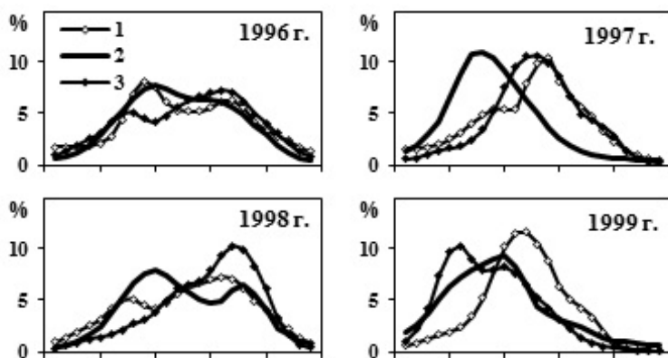
Рис. 4.9 а. Динамика ската молоди и возврата производителей горбуши на о-в Кунашир в 1996–1999 гг. (указан год возврата поколения): 1 – скат молоди, 2 – возврат этого поколения, 3 – последующий скат молоди дочернего поколения.
