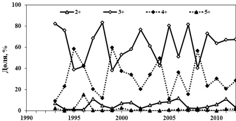
Рис. 3.9. Динамика возрастного состава кеты в р. Илюшина в 1993–2012 гг.
