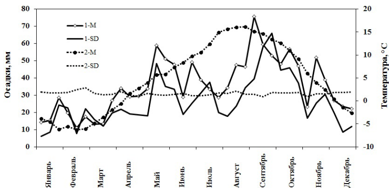
Рис. 2.1. Декадная динамика количества осадков и температуры воздуха (М и SD) на о-ве Кунашир, по данным СУГМС в среднем за 1969–1979 гг.: 1 – осадки, 2 – температура.
