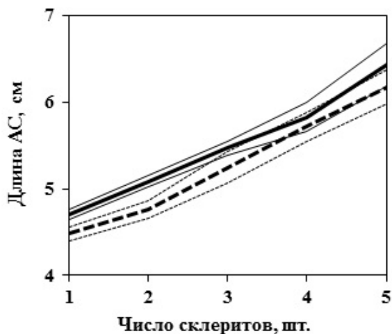
Рис. 5.3. Изменения длины тела в зависимости от числа склеритов на чешуе у молоди кеты о-ва Итуруп – на прибрежном морском мелководье в районе впадения рек Курилка и Рыбацкая (сплошная линия) и в протоке оз. Сопочное (пунктирная линия) – в среднем в 1984, 1986–1988 гг.: тонкими линиями показаны границы 95-процентного доверительного интервала.
