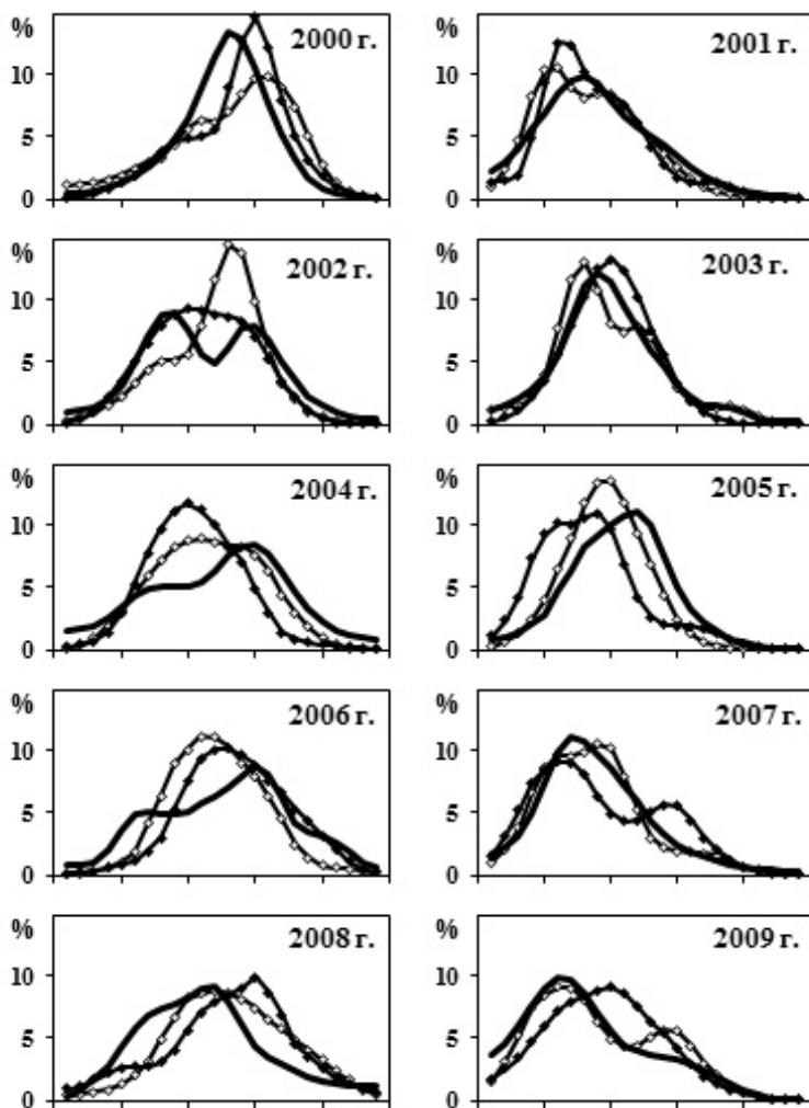
Рис. 4.9 б. Динамика ската молоди и возврата производителей горбуши на о-в Кунашир в 2000–2009 гг. (указан год возврата поколения): 1 – скат молоди, 2 – возврат этого поколения, 3 – последующий скат молоди дочернего поколения.
