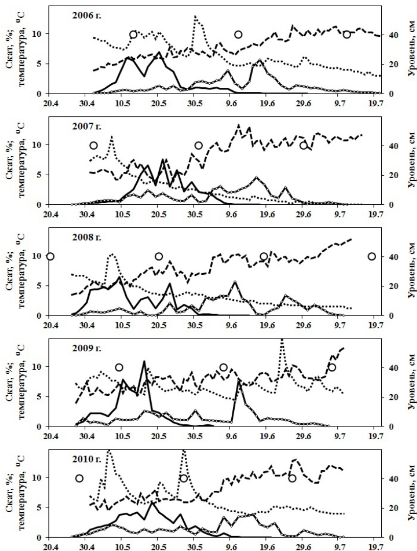
Рис. 3.13 б. Динамика покатной миграции молоди горбуши (1) и кеты (2), температуры (3) и уровня воды (4) в р. Илюшина в разные годы: 5 – дата полнолуния.
