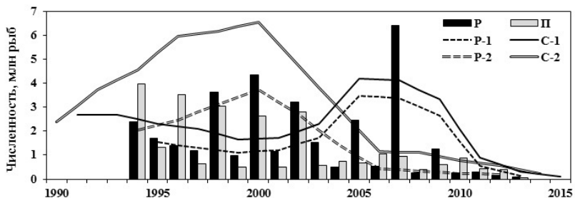
Рис. 4.7. Количественное соотношение ранней (P) и поздней (Ф) форм горбуши в возвратах горбуши на о-в Кунашир в 1994–2013 гг.: линии – скользящие средние, рассчитанные по трем смежным значениям; P-1 и P-2 – численность ранней формы, C-1 и C-2 – суммарная численность обеих форм в нечетные (1) и четные (2) годы, соответственно.
