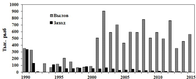
Рис. 3.18. Уловы кеты в водах Кунашира и величина заходов производителей в реки и озера острова в 1990–2015 гг. (1992, 1993, 2015 гг. – нет данных по заходам).
