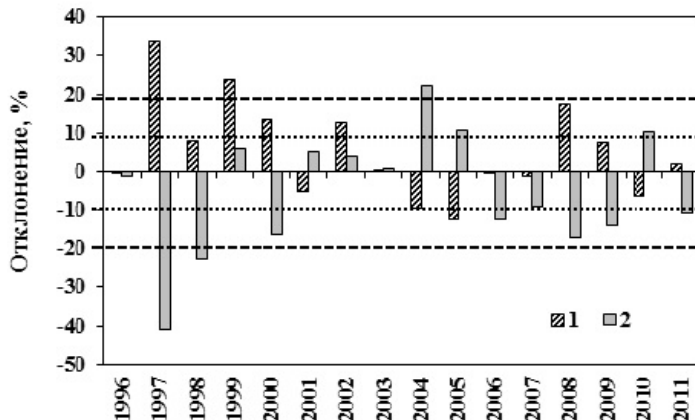
Рис. 4.10. Изменения в поколениях горбуши 1996–2011 гг. (по году возврата) разницы в доле ранних мигрантов при сопоставлении ската молоди с последующим возвратом рыб (1) и затем этого возврата производителей со скатом дочернего поколения (2): пунктиром показаны границы распределения значений для диапазона \pm 0,5SD , штрихом – для \pm SD .
