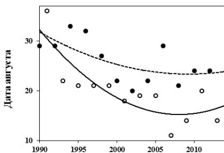
Рис. 4.1. Изменения даты достижения 50-процентной кумуляты вылова горбуши на о-ве Кунашир в нечетные (светлые символы, сплошная линия) и четные (темные символы, пунктирная линия) 1991–2013 гг.
