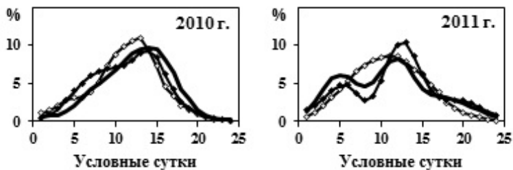
Рис. 4.9 в. Динамика ската молоди и возврата производителей горбуши на о-в Кунашир в 2010–2011 гг. (указан год возврата поколения): 1 – скат молоди, 2 – возврат этого поколения, 3 – последующий скат молоди дочернего поколения.
