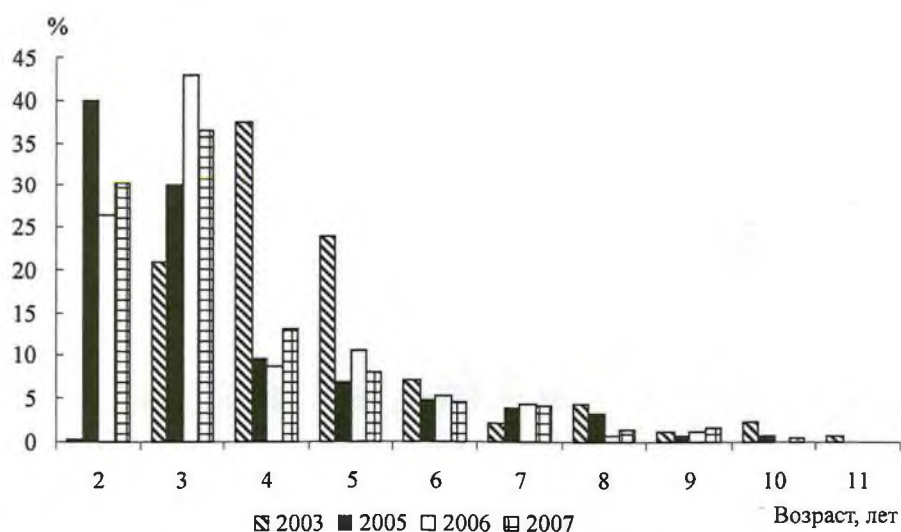
Рис. 5. Возрастная структура наваги зал. Одян за 2003–2007 гг.
