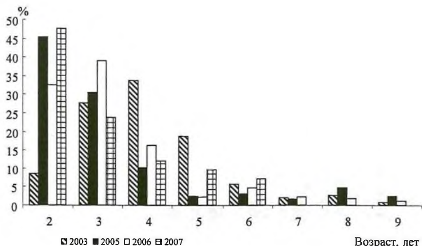
Рис. 4. Возрастная структура наваги бух. Гертнера в 2003–2007 гг.
