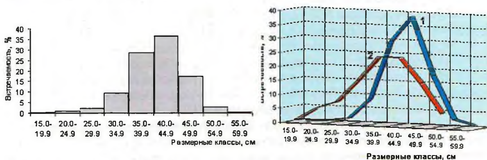
Рис. 7. Общий размерный состав уловов желтобрюхой камбалы (слева) и на различных участках побережья (справа): 1 – Притауйский район; 2 – зал. Одян
