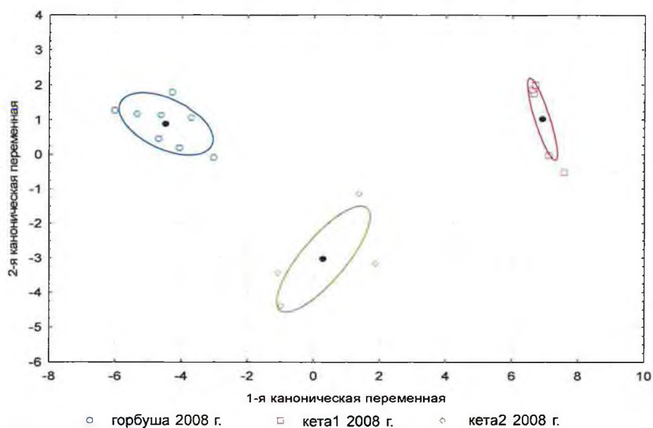
Рис. 7. Взаиморасположение выборок кеты и горбуши в плоскости главных канонических переменных
