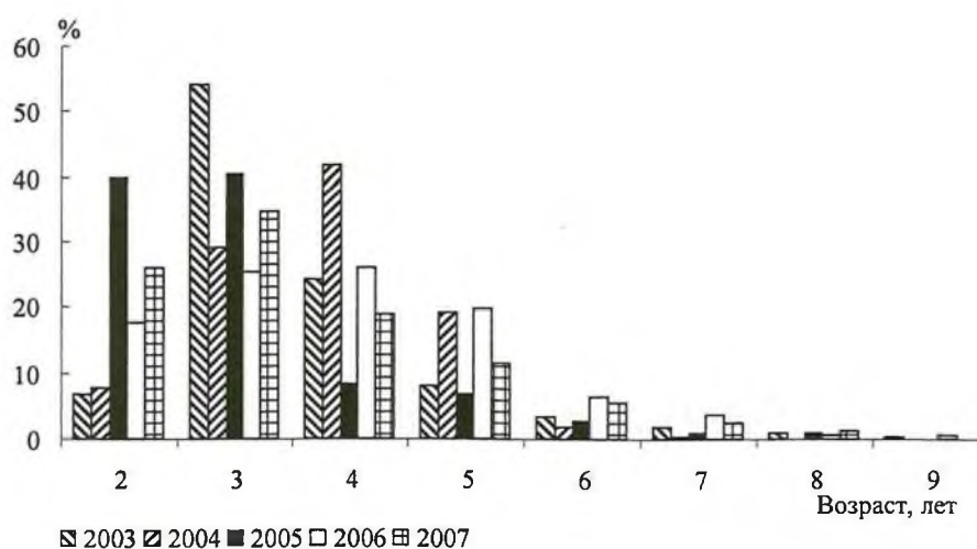
Рис. 3. Возрастная структура наваги Мотыклейского залива в 2003–2007 гг.
