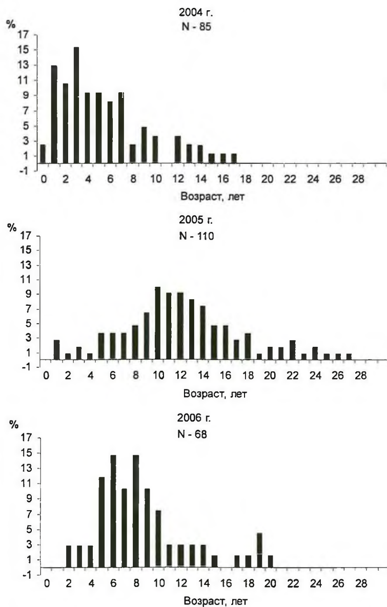
Рис. 6. Возрастная структура ларги, добытой в Таймырской губе в октябре-ноябре 2004–2006 гг.
