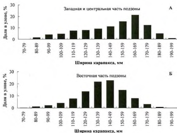
Рис. 2. Размерный ряд самцов равношипного краба в западной, центральной (А) и восточной (Б) частях Северо-Охотоморской подзоны
