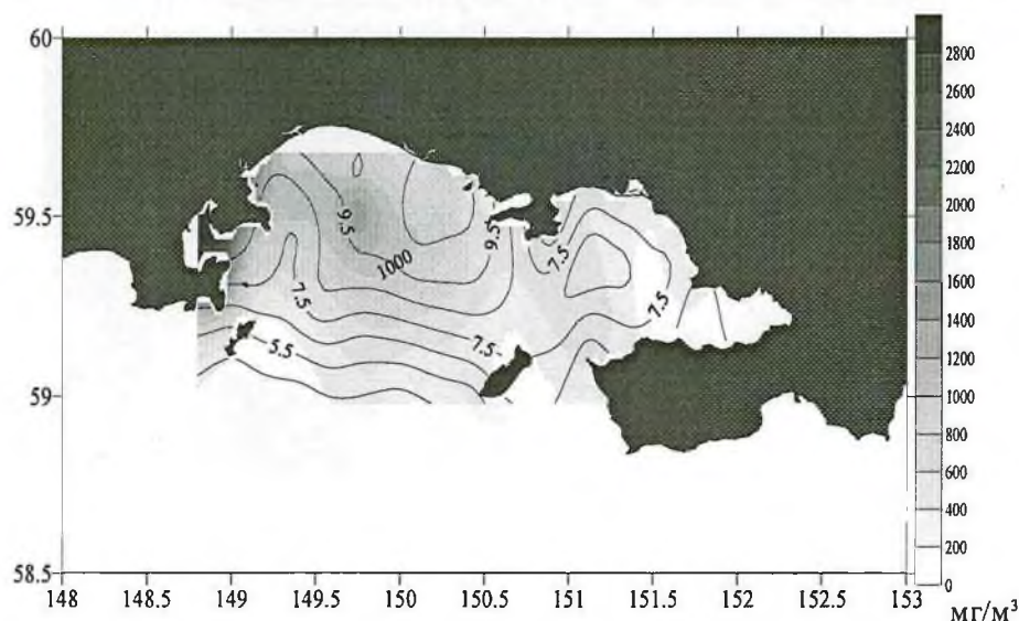
Рис. 9. Распределение температуры воды ( ^\circ\text{C} ) на поверхности и биомассы зоопланктона ( \text{мг}/\text{м}^3 ) в Тауйской губе в 2004 г.
