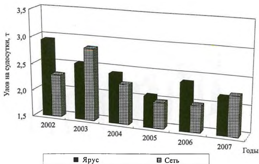
Рис. 7. Динамика уловов черного палтуса на судосутки в 2002–2007 гг.
