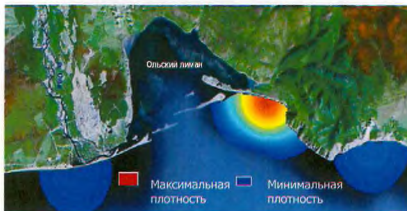
Рис. 7. Плотности распределения наваги на модельном полигоне в июне-июле 2008 г.
