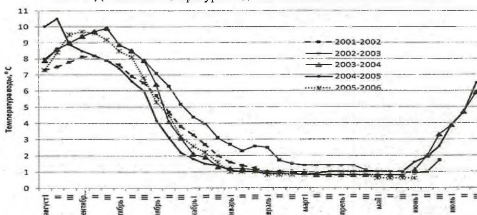
Рис. 2. Динамика температуры воды на Арманском ЛРЗ в 2002–2006 гг.
