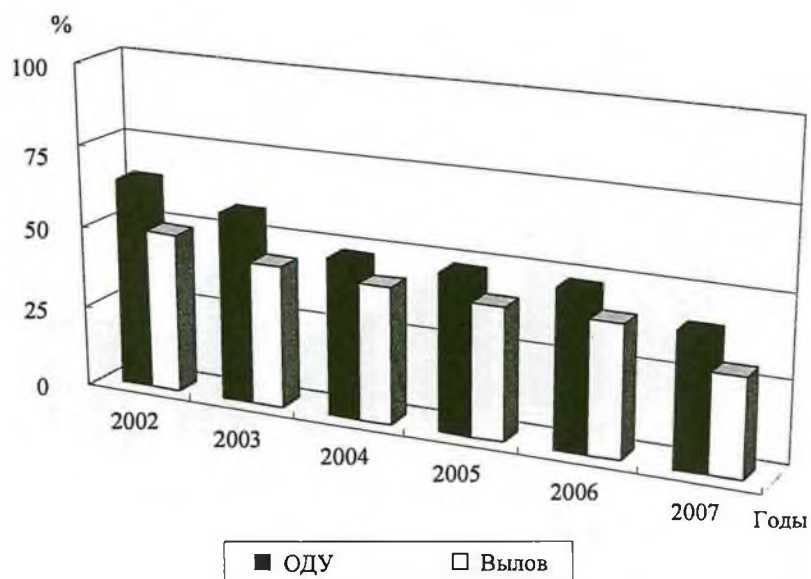
Рис. 5. ОДУ и вылов черного палтуса в Северо-Охотоморской подзоне в 2002–2007 гг. (в % от ОДУ 2000 г.)
