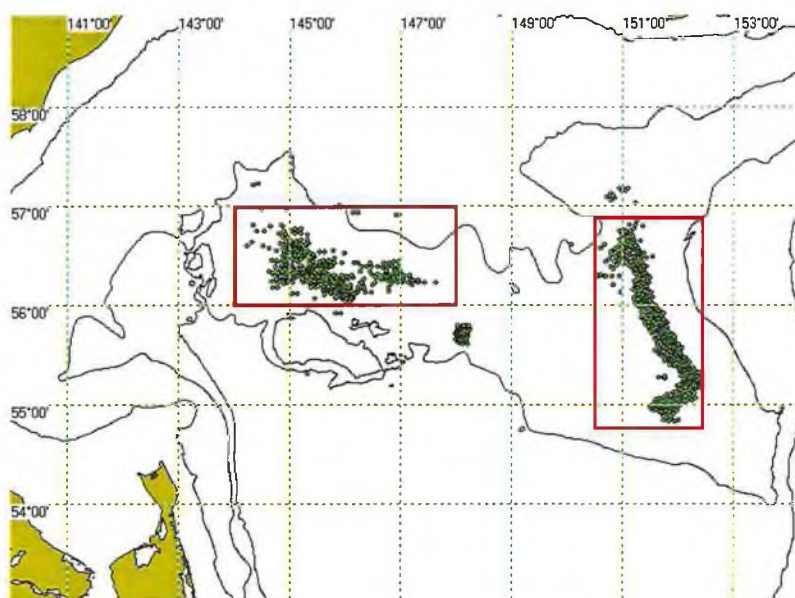
Рис. 1. Скопления равношипного краба промыслового размера по данным 2005 г.
