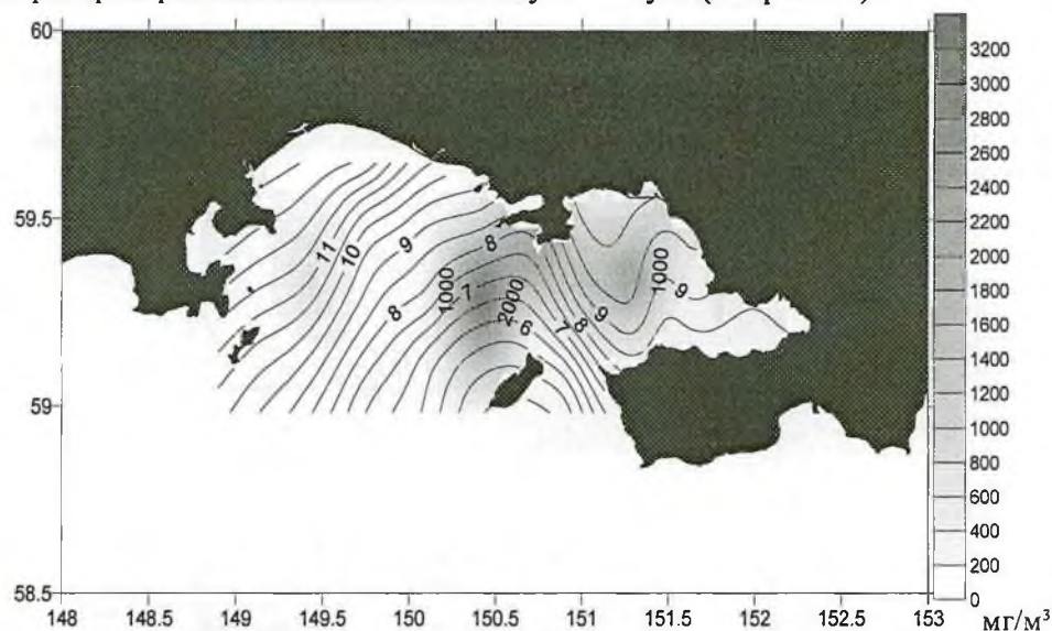
Рис. 10. Распределение температуры воды на поверхности (°C) и биомассы зоопланктона (мг/м³) в Тауйской губе в 2005 г.
