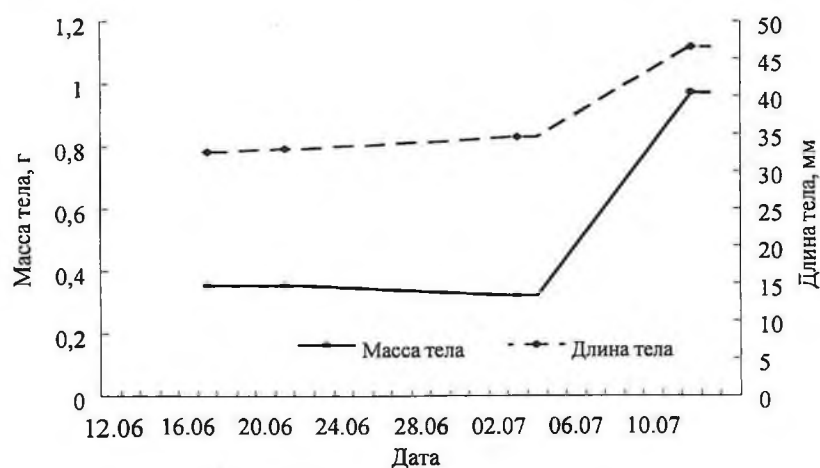
Рис. 3. Изменение длины и массы тела молоди кеты в процессе подращивания в условиях оз. Глухое в 2007 г.
