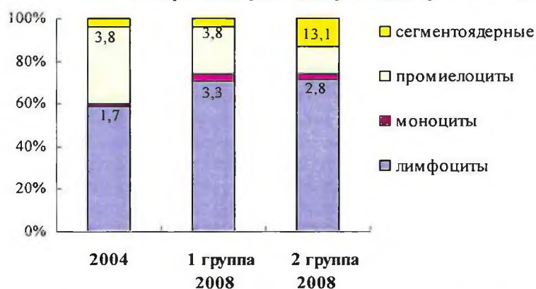
Рис.10. Соотношение форм лейкоцитов в крови молоди кеты из устья р.Ола в 2004 и 2008 гг.
