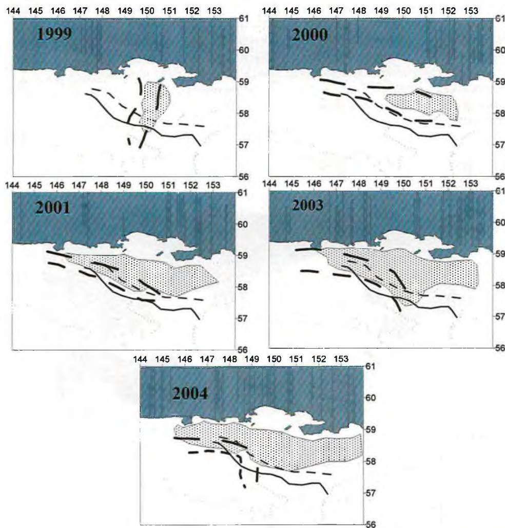
Рис. 6. Положение границ фронтальных зон в сентябре по годам относительно средне-многолетнего сентябрьского положения в Притауйском районе в периоды: 1999 г. – сентябрь 2 декада; 2000 г. – сентябрь 2, 3 декады; 2001 г. – сентябрь 3 декада, октябрь 1 декада; 2003 г. – сентябрь 2, 3 декады; 2004 г. – сентябрь 3 декада, октябрь 1 декада
