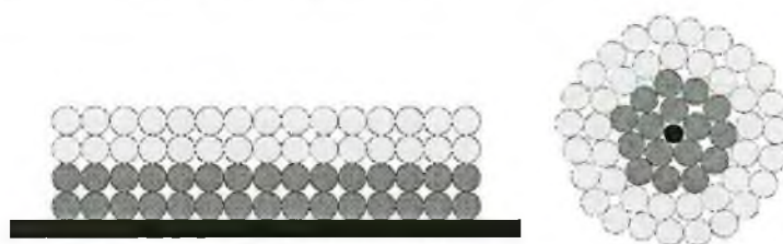
Рис. 3. Схема поперечного разреза кладки икры на плоском (слева) и цилиндрическом субстрате (справа). Темным выделены икринки, расположенные в зоне риска
