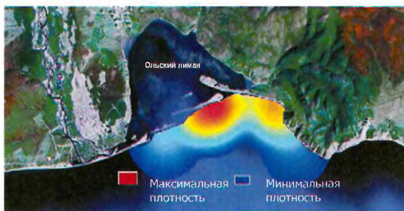
Рис. 5. Плотности распределения молоди кеты на модельном полигоне в июне-июле 2008 г.
