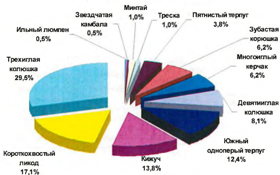
Рис. 3. Доли фоновых видов рыб в уловах
