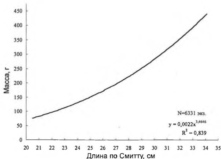
Рис. 5. Зависимость массы производителей охотской сельди от длины тела
