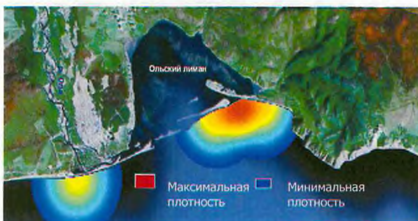
Рис. 9. Плотности распределения молоди мойвы на модельном полигоне в июне-июле 2008 г.
