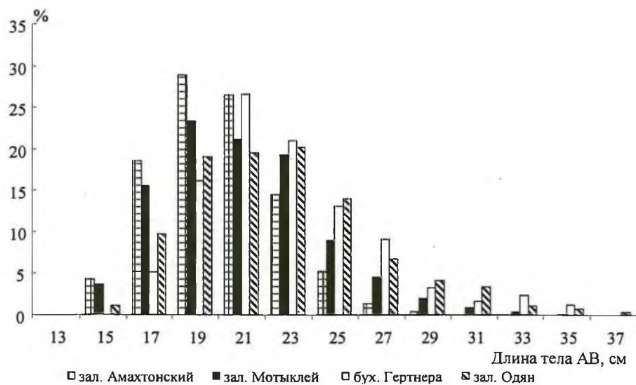
Рис. 6. Размерная структура наваги по средним показателям совокупной выборки из различных районов промысла в Тауйской губе за 2002–2007 гг.
