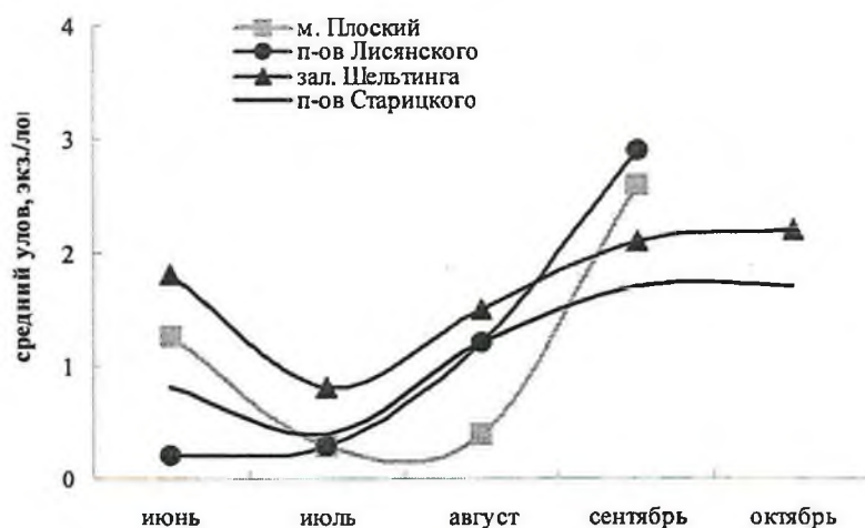
Рис. 3. Динамика среднемноголетних уловов колючего краба по районам исследований
