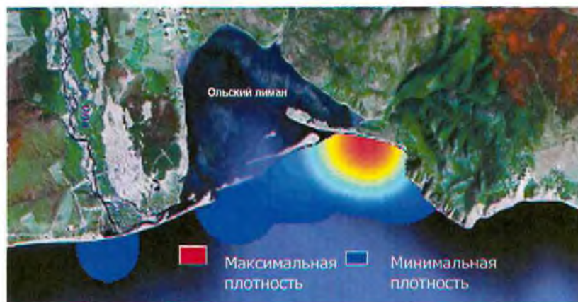
Рис. 6. Плотности распределения сельди на модельном полигоне в июне-июле 2008 г.
