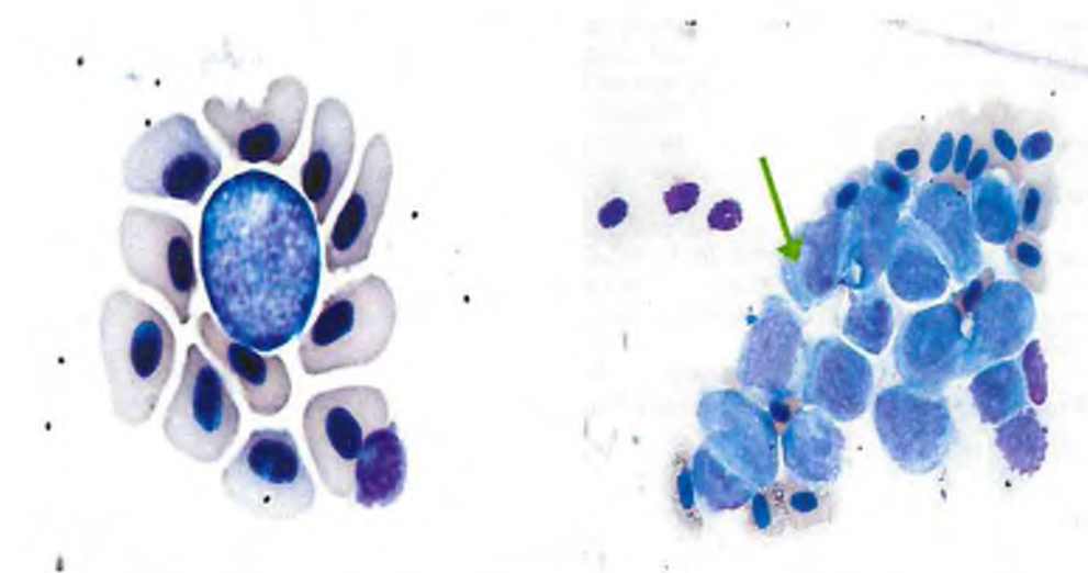
Рис. 10. Гемогистобласты на мазках крови молоди горбуши из устья р. Ола
