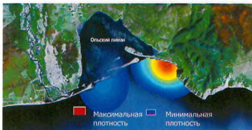
Рис. 8. Плотности распределения малоротой корюшки на модельном полигоне в июне-июле 2008 г.
