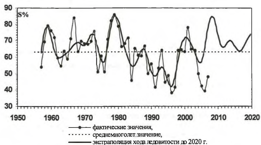
Рис. 1. Многолетний ход среднезимних (январь–апрель) значений ледовитости (S%) Охотского моря (Устинова и др., 2002)
