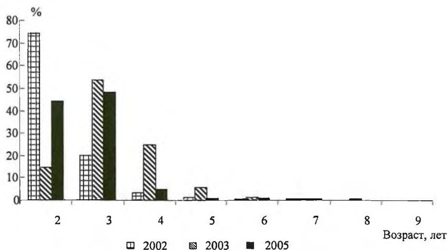
Рис. 2. Возрастная структура наваги залива Амахтонский за ряд лет
