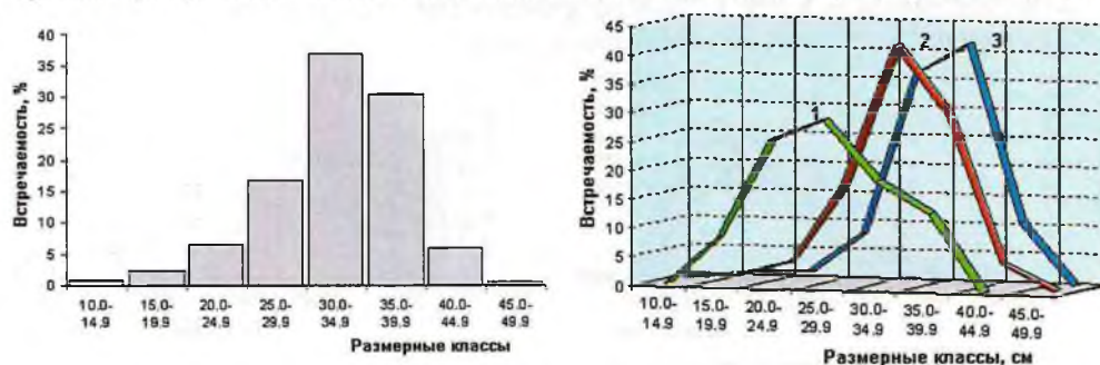
Рис. 2. Общий размерный состав уловов желтоперой камбалы (слева) и на различных участках побережья (справа): 1 – бух. Нагаева; 2 – Тауйская губа; 3 – Притауйский район
