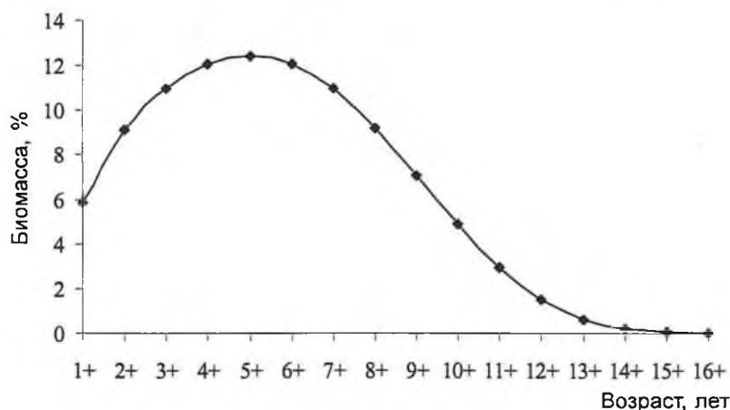
Рис. 1. Доля биомассы поколений в общей биомассе популяции трески северной части Охотского моря
