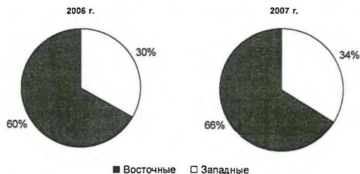
Рис. 1. Распределение производителей охотской сельди по группам нерестилищ
