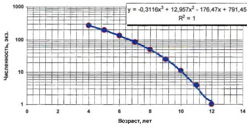
Рис. 2. Номограмма убывающей кривой хариуса по возрастам
