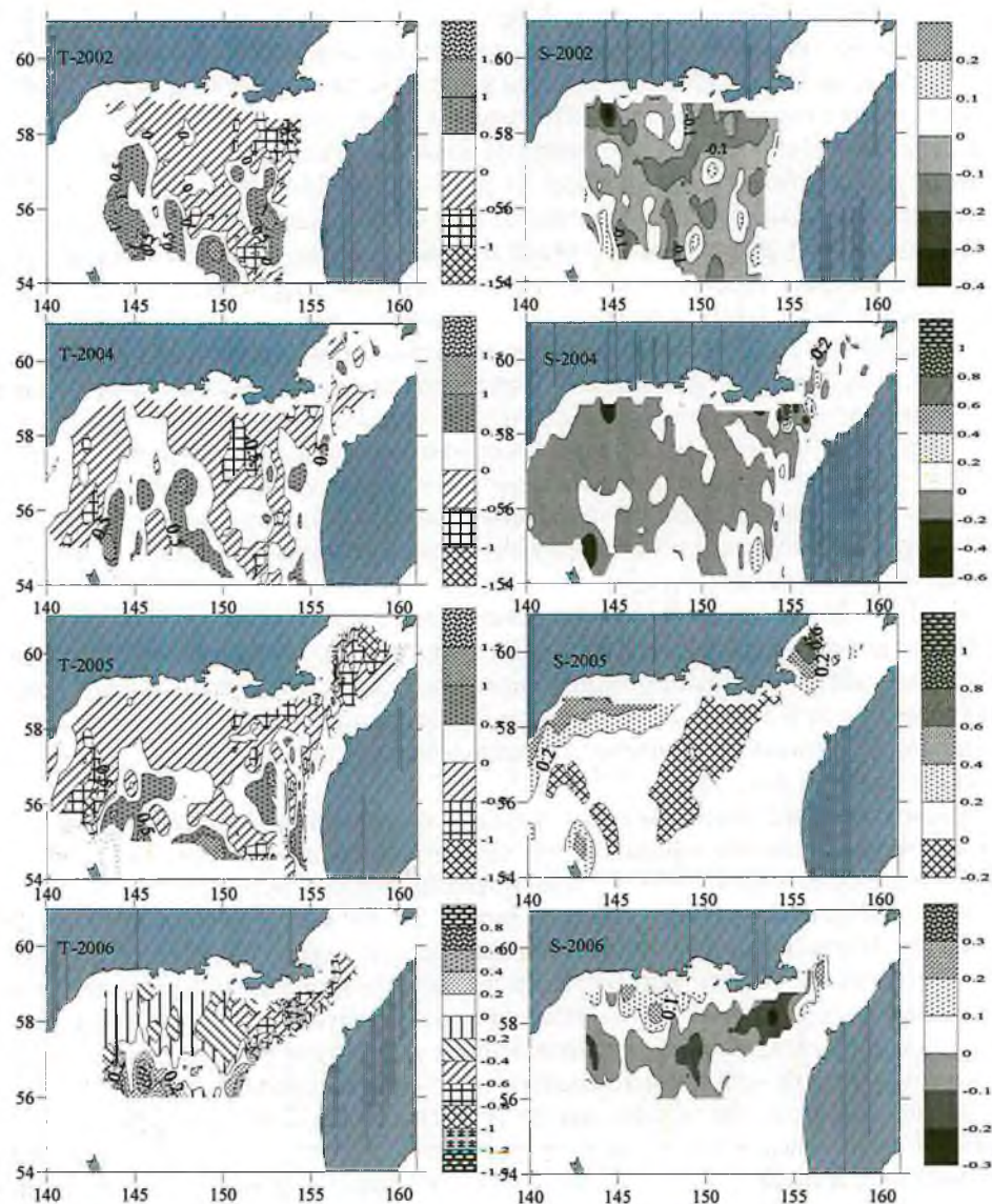
Рис. 4. Распределение аномалий температуры (левый столбец) и солёности (правый столбец) на горизонте 100 м с 2002 по 2006 гг.
