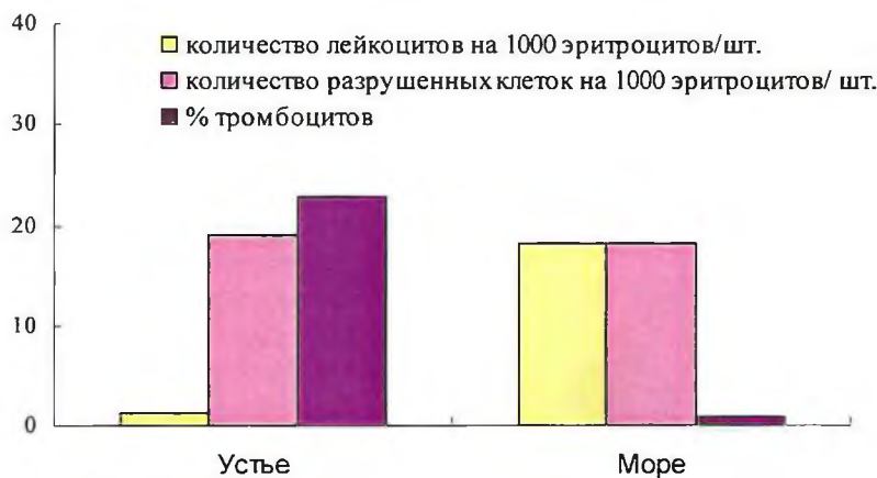
Рис. 5. Доля тромбоцитов, количество лейкоцитов и разрушенных клеток на мазках крови молоди горбуши из участков Ольского лимана с различной солёностью в 2008 г.
