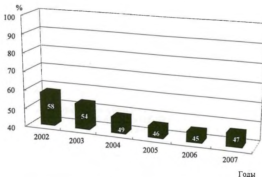
Рис. 2. Доля самок черного палтуса в уловах в 2002–2007 гг., %
