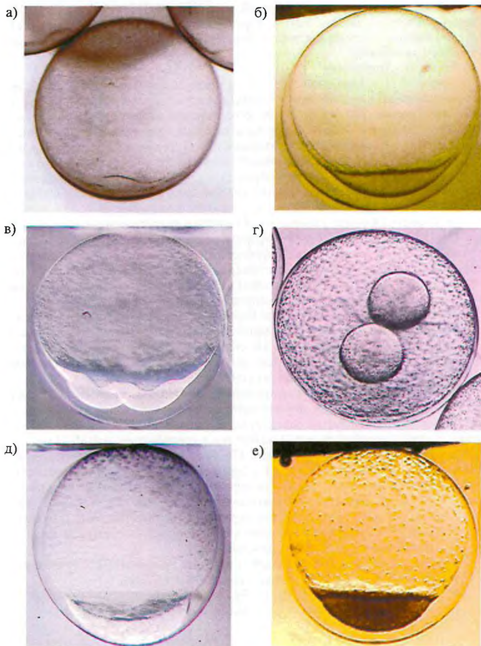
Рис. 1. Эмбриональное развитие полярной камбалы: а – оплодотворенная икринка, на анимальном полюсе в яичевой оболочке имеется воронковидное углубление микропиле; б – цитоплазматический бугорок (бластодиск) на анимальном полюсе яйца (возраст 10 часов); в – два бластомера (возраст 11 часов); г – то же, вид сверху, со стороны вегетативного полюса; д – ранняя бластула (возраст 42 часа); е – поздняя бластула, в основании бластулы виден светлый слой перибласта (возраст 66 часов)
