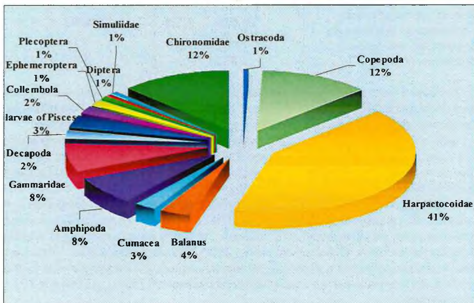
Рис. 2. Спектр питания молоди кеты в Ольском лимане Тауйской губы в 2004 г. (А) и в 2005 г. (Б) (% от общего количества экземпляров)
