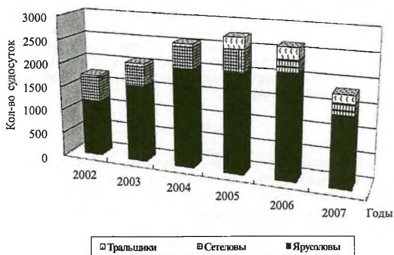
Рис. 6. Количество судосудок на лову ярусоловов, сетелювов и тральщиков на промысле черного палтуса в 2002–2007 гг.
