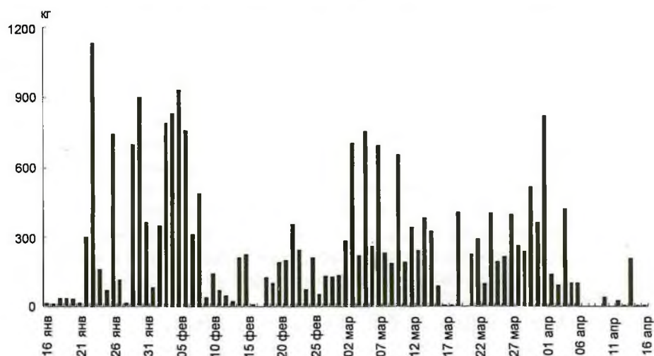
Рис. 1. Суточная динамика вылова наваги в Таймской губе по среднееголетним данным на примере зал. Амахтонский
