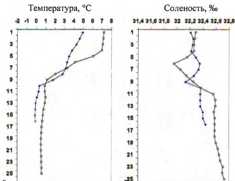
Рис. 14. Вертикальное распределение температуры и солёности в районе нерестилищ сельди (бух. Светлая и Нагаева)
