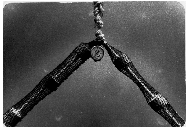
Рисунок 17. Фрагмент коллектора непрерывного (пилообразного) в воде, цилиндры из пенопласта обшиты сетной оболочкой
