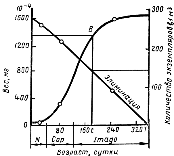
Рис. 1. Рост элиминации рачка Acanthodiaptomus denticornis .
