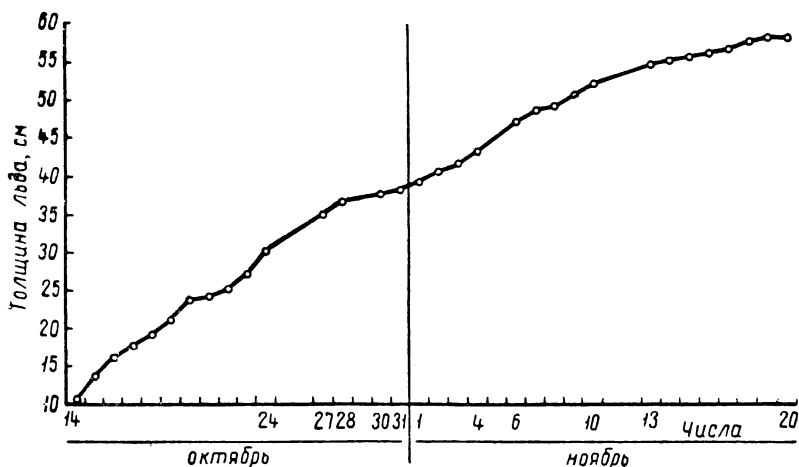
Скорость увеличения ледового покрова на оз. Муосталах в 1958 г.
