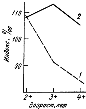
Относительный вес печени озерного голяна (1971 г.) 1 — опыт; 2 — контроль.
